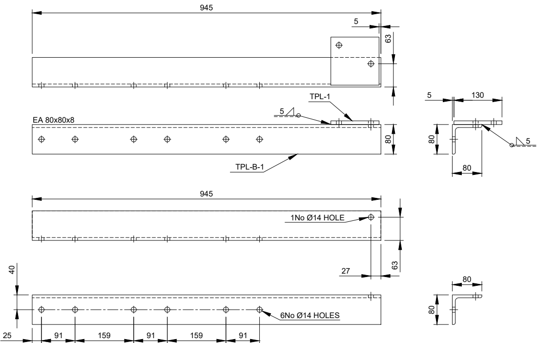
TPL-B-1 - EA 80x80x8 Scale 1:10
